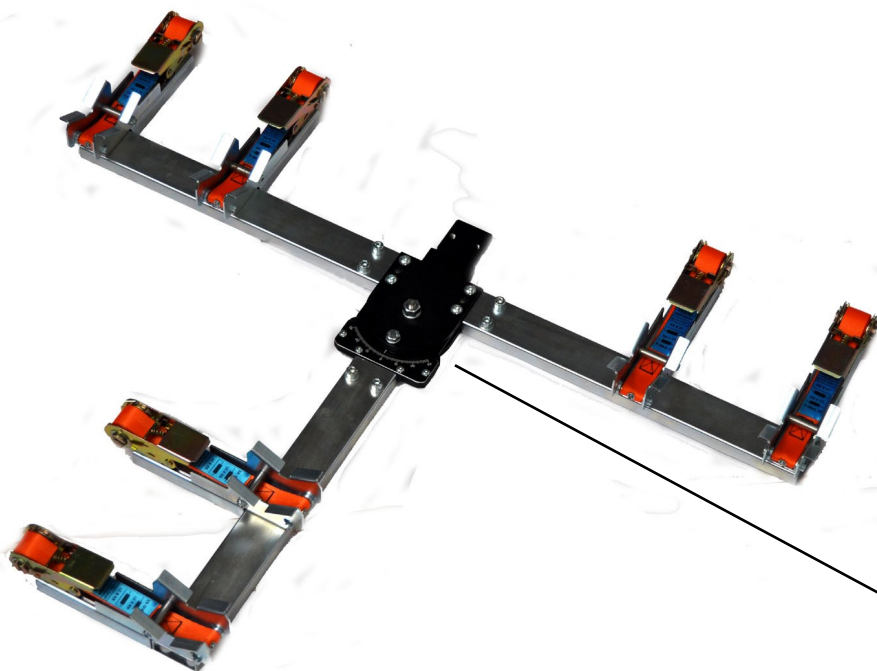
Versione con dispositivo SRC ( a richiesta) SRC regulation system version (on request)
